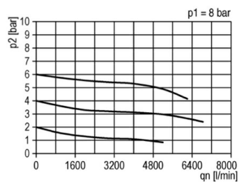
Průtokový diagramm
