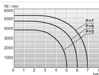
Průtokový diagramm 1/2"
