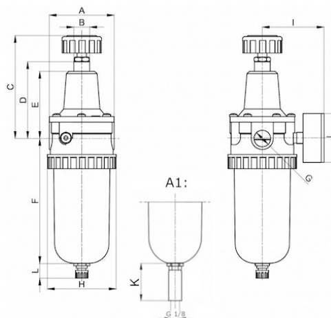
A1: automatický vypouštěcí ventil
