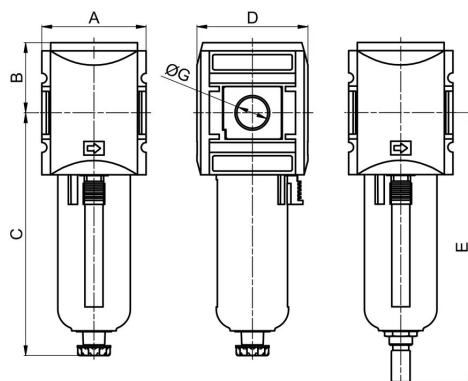
poloautomatický vypouštěcí ventil
